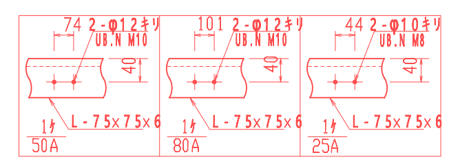
ボルト穴詳細
